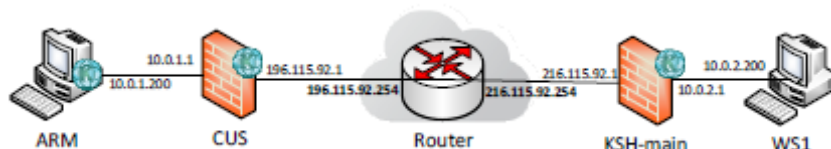
Рис. 1 Сетевая среда по условию задания
