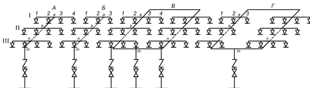
Рисунок Б.1 - Расположение оросителей на распределительной сети
