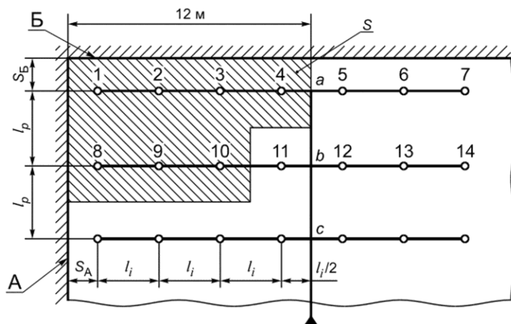
Рисунок 6.1. Устройство несоосного перехода труб
